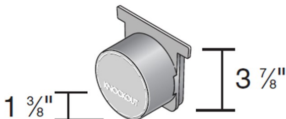
#713 END OUTLET
